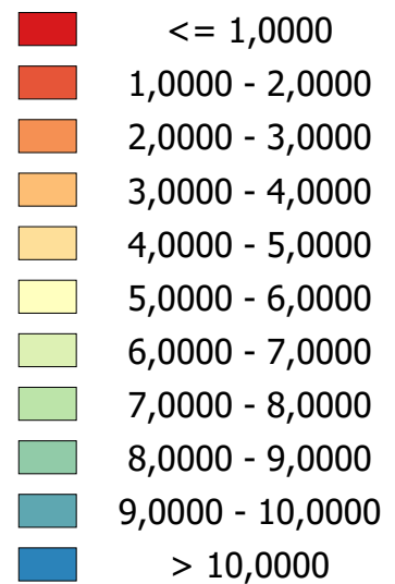
VIENTOS 80 M JUNIO BOLIVAR (m/s)
